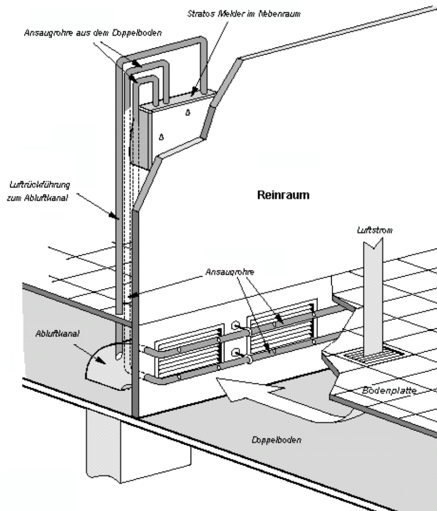
Bild 3 Primäre Ansaugung mit Luftrückführung in den Reinraum
