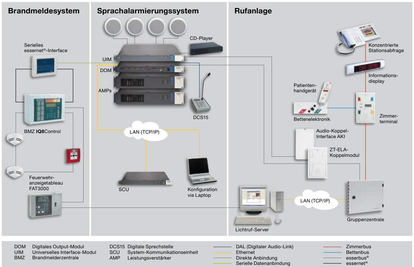
Prinzipialschaltung für die Anbindung von Sprachalarmierungskomponenten an die Gewerke Brandmeldetechnik und Pflegekommunikation
