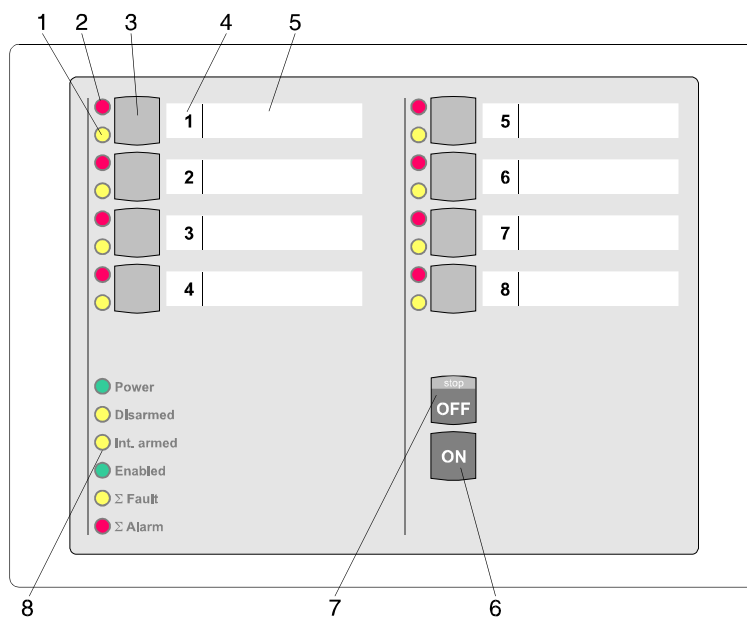
Abb. 29 Bedienteil 012532
