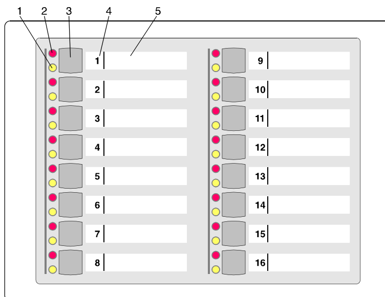
Abb. 31 Bedienteil 012542
