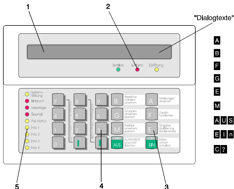
Abb. 8 Bedienteil 012540/012541
