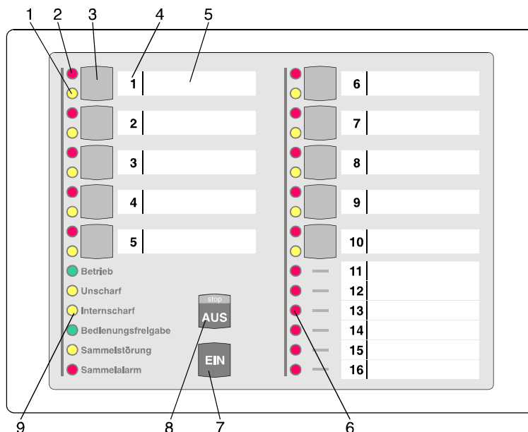
Abb. 25 Bedienteil 012544
