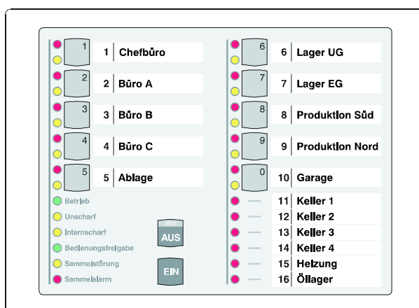
Abb. 26 Code-Ziffernbelegung auf den Sperrtasten
